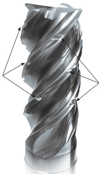
Detail přerušovaného břitu - obvodové drážky ve spirále
