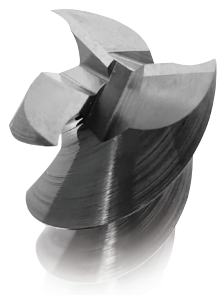
Detail břitu
