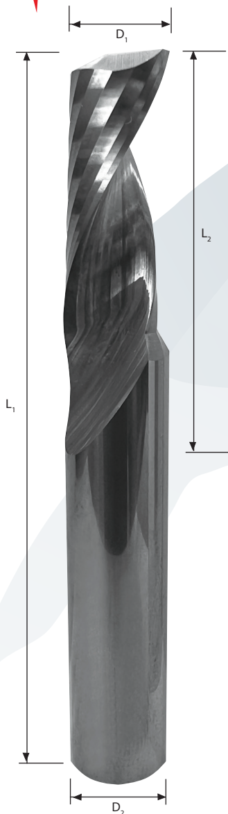
Detail břitu
