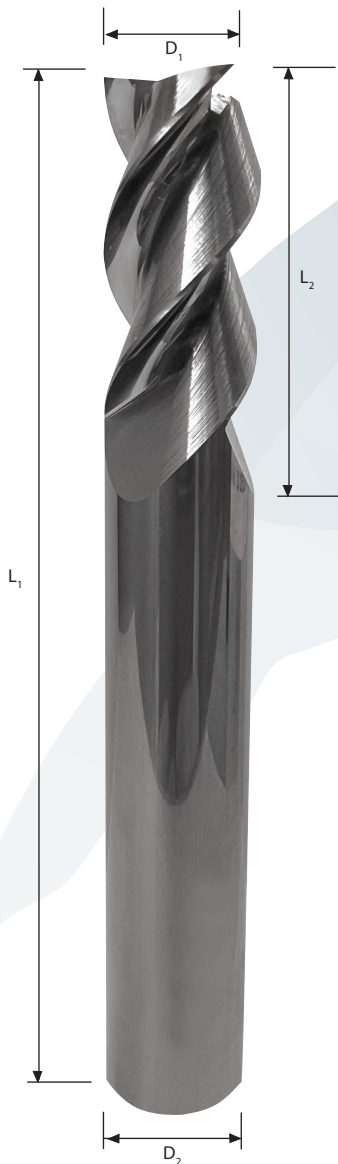
Detail břitu
