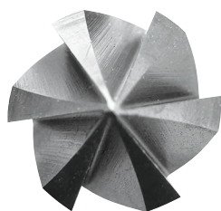
Detail břítu
